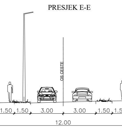
POPREČNI PRESJEK CESTE 1:200
