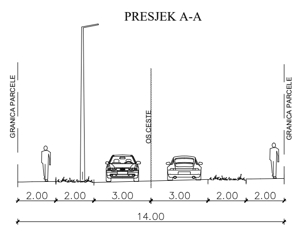
POPREČNI PRESJEK CESTE 1:200
