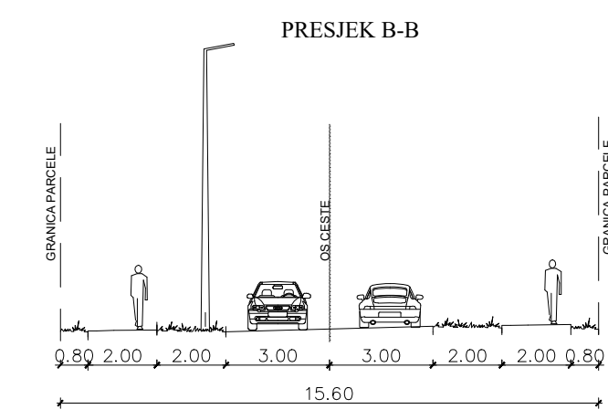
POPREČNI PRESJEK CESTE 1:200
