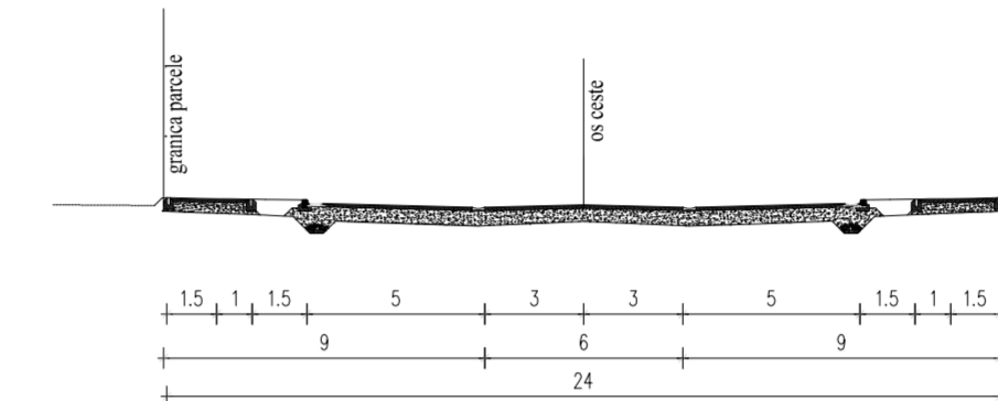
KARAKTERISTIČNI POPREČNI PRESJEK A - A
