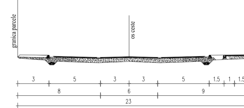
KARAKTERISTIČNI POPREČNI PRESJEK B - B
