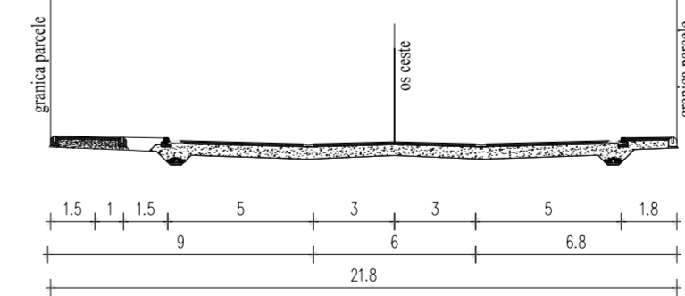
KARAKTERISTIČNI POPREČNI PRESJEK D - D
