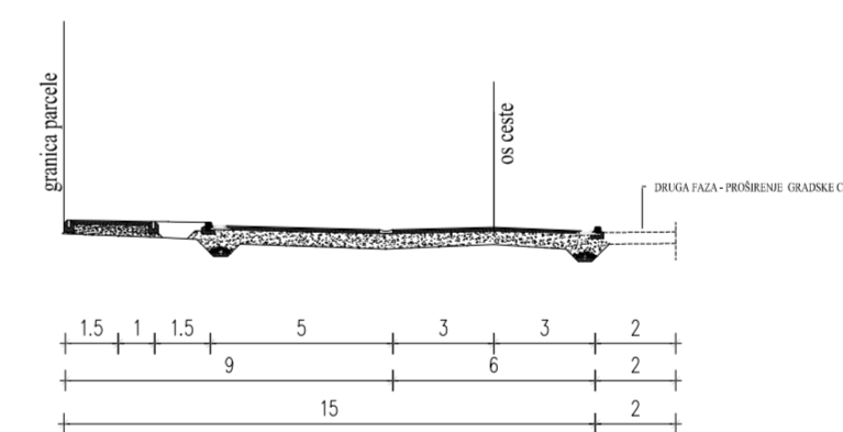
KARAKTERISTIČNI POPREČNI PRESJEK C - C
